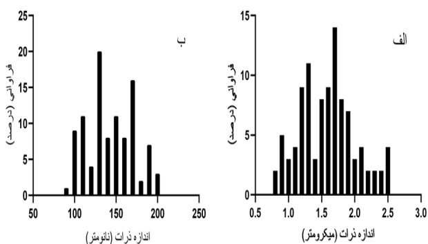
شکل ۳: توزیع اندازه ذره ای میکروذرات (الف) و نانوذرات اکسید روی (ب) که نشان دهنده پراکنش ذرات در دامنه اندازه های میکرومتر و نانومتر می باشد.
