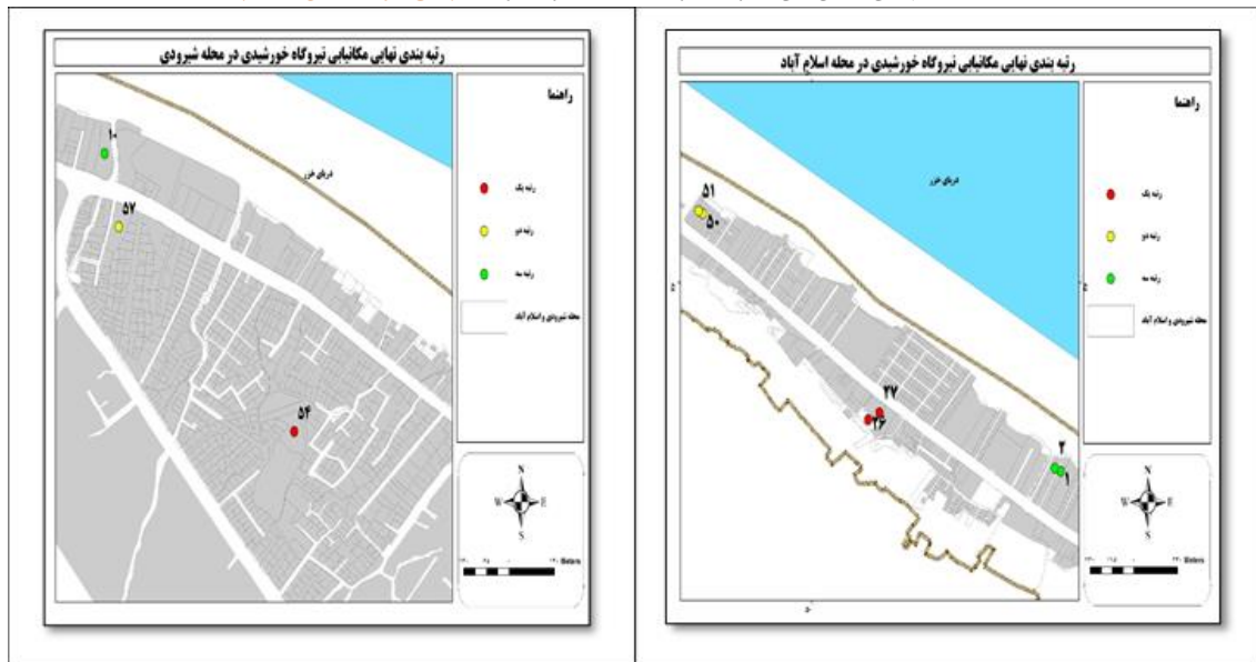
شکل ۵. نقاط نهایی مکان‌یابی نیروگاه خورشیدی در نمونه موردی (منبع: نویسندگان، ۱۴۰۳)
