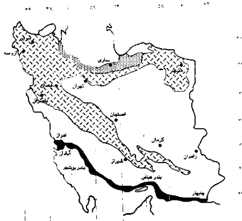
تقسیمات اقلیمی روی نقشه ایران
