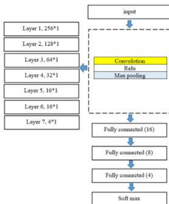
شکل (۳): شبکه عصبی کانولوشنی طراحی شده در این مطالعه
