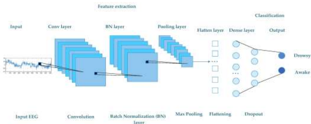
شکل (۲): نمودار شبکه عصبی کانولوشنی پیشنهادی [۲۸]
