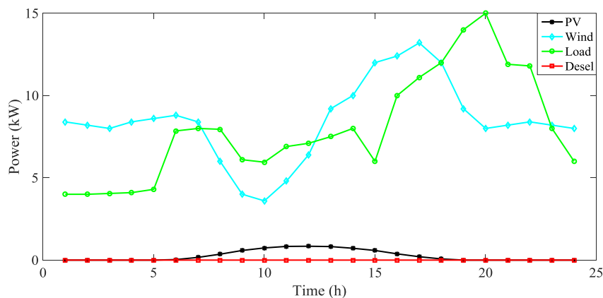
شکل (۱۰): منحنی روزانه توان تولیدی دیزل ژنراتور، واحد بادی و فتوولتاییک در مورد مطالعاتی چهارم Figure (10): Daily power output curve of diesel generator, wind and photovoltaic unit for the fourth case study
