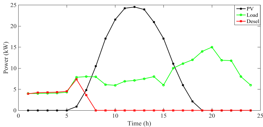
شکل (۹): منحنی روزانه توان تولیدی دیزل ژنراتور، واحد بادی و فتوولتاییک در مورد مطالعاتی سوم Figure (9): Daily power generation curve of diesel generator, wind and photovoltaic unit for the third case study
