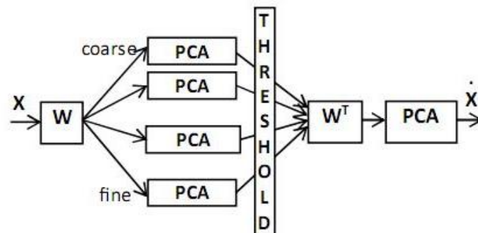
شکل (۱): مراحل مختلف الگوریتم MSPCA [۱۴]
