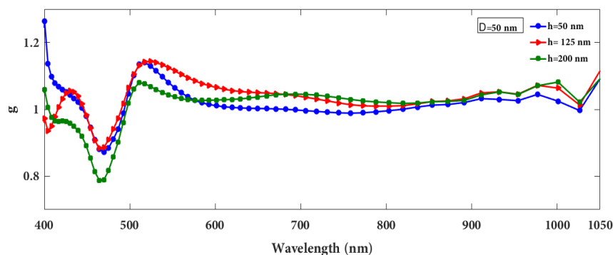
شکل (۱۰): ضریب افزایش (g) با ارتفاع متفاوت نانوذرات استوانه‌ای نقره در D = 50nm Figure (10): The enhancement ratio g(λ) with different height of cylindrical Ag NPs at D=50 nm
