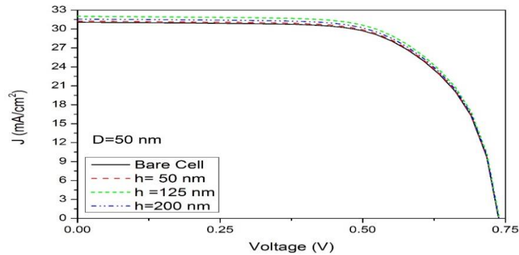
شکل (۱۱): منحنی‌های J-V محاسبه شده برای سلول‌های خورشیدی لخت (خط پیوسته) و پلاسمونی CIGS توسط نانوذرات استوانه‌ای نقره با D = 50nm در ارتفاع متفاوت
