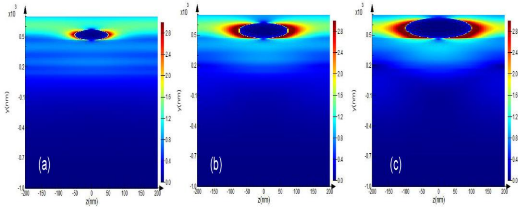
شکل (۷): محاسبه پروفایل‌های جذب شده توسط FDTD برای سلول‌های خورشیدی CIGS که توسط نانوذرات کروی نقره با قطر (a) ۱۰۰ نانومتر، (b) ۱۵۰ نانومتر و (c) ۲۰۰ نانومتر در \lambda=575 nm مرتب شده‌اند
