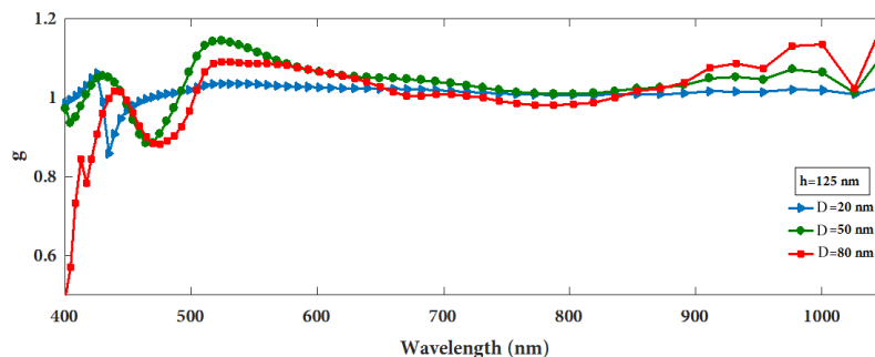
شکل (۱۲): نسبت افزایش g(\lambda) با قطرهای مختلف نانوذرات استوانه‌ای، در h=125\text{nm}
