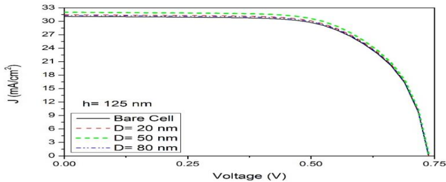
شکل (۱۴): منحنی J - V سلول‌های خورشیدی لخت (خط پیوسته) و پلاسمونی CIGS با نانوذرات نقره‌ای استوانه‌ای با h=125 nm در قطرهای مختلف
