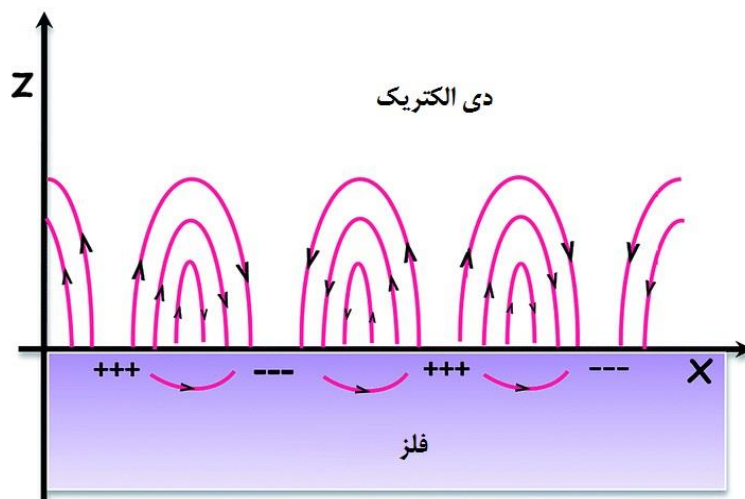
شکل (۲): برانگیزش یک موج پلاسماوی سطحی در فصل مشترک بین یک فلز با ثابت دی‌الکتریک \epsilon_2 و یک جسم دی‌الکتریک یا خلأ با ثابت دی‌الکتریک \epsilon_1
