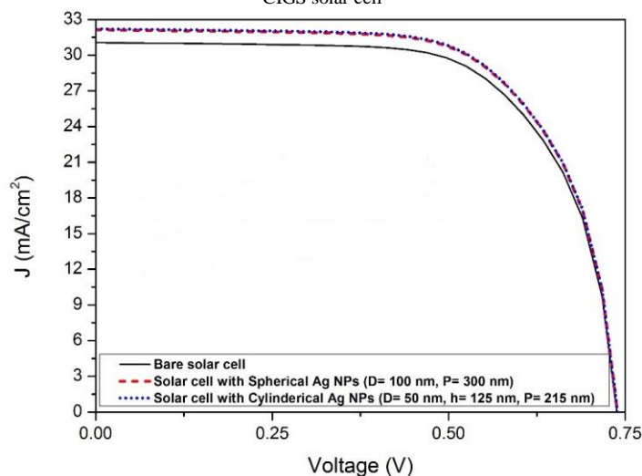
شکل (۱۶): منحنی‌های J - V سلول خورشیدی CIGS بدون نانوذرات و با نانوذرات نقره کروی و استوانه‌ای
