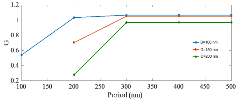
شکل (۸): تغییر فاکتور افزایش G با دوره تناوب قطرهای مختلف نانوذرات کروی
