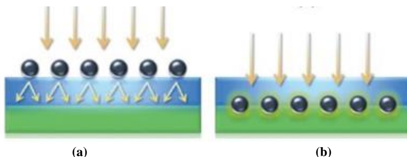
شکل (۳): (a) به دام افتادن نور توسط نانوذرات فلزی و پخش با زوایای مختلف و افزایش عمق مؤثر، (b) قرار گرفتن نانوذرات فلزی درون نیمه‌هادی و برانگیخته شدن میدان نزدیک ذره و تولید زوج الکترون-حفره
