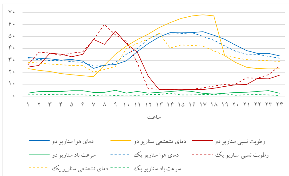
شکل ۷: نتایج شبیه سازی نرم افزار انویمت در خصوص دو سناریو اول و دوم
