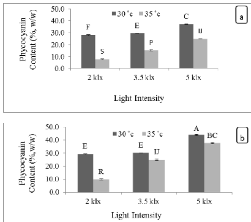
شکل 1- مقادیر تولید فایکوسیانین (% w/w) با استفاده از گلوکز در شدت نورهای مختلف و دو محیط کشت بچ (a) و فدبج (b) شرایط
