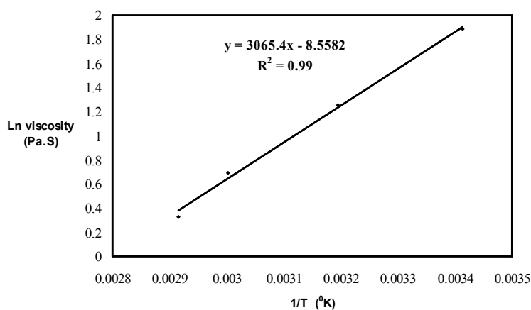
شکل ۲- اثر دما بر ویسکوزیته‌ی خمیر خرما
