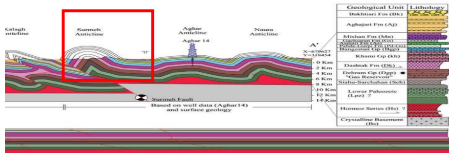
شکل ۷- قسمتی از مقطع عرضی در امتداد AA' از منطقه کوه سورمه از نقشه شکل ۶
