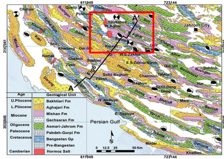
شکل ۶- نقشه زمین شناسی جنوب غرب فارس - کادر قرمز رنگ منطقه کوه سورمه و سازندهای اصلی آن.
