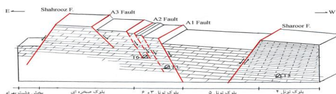
شکل ۸- شماتیک گسل های اصلی عمود بر محور تاقدیس کوه سورمه
