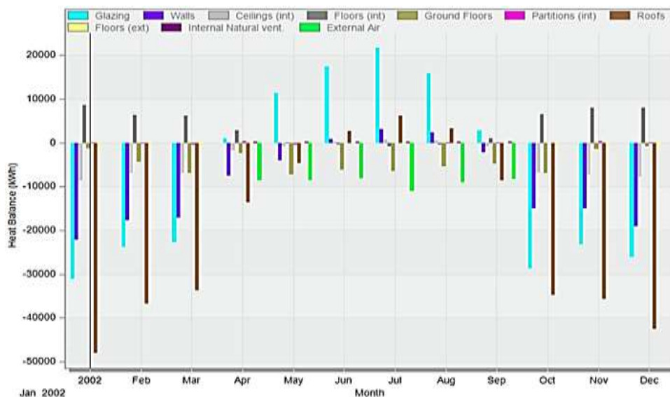
شکل ۹- نمودار وضعیت انتقال حرارت سطوح در وضعیت فعلی
