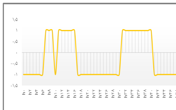
شکل ۱۲- زمان‌های شارژ و دشارژ شدن باتری‌ها در حالت مدیریت سمت تقاضا
