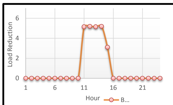
شکل ۲۲- میزان مشارکت ریزشکه در باس ۵
