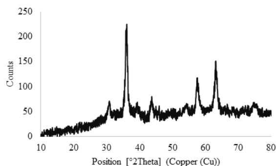
شکل ۱۱ الگوی XRD نانوکاتالیست \text{Fe}_3\text{O}_4@\text{PDBOA}-\text{Cu}
