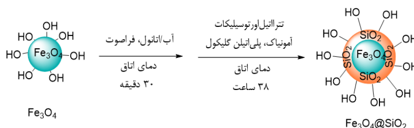
شکل ۱ طرحواره سنتز نانوذره های مغناطیسی Fe_3O_4 پوشینه دار شده با سیلیکا
