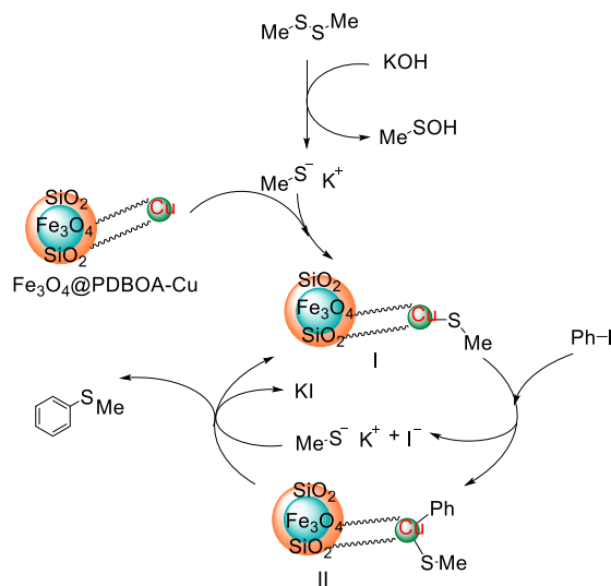
شکل ۱۷ طرح‌واره سازوکار پیشنهادی تبدیل DMDS به MPS در حضور کاتالیست \text{Fe}_3\text{O}_4@\text{PDBOA-Cu}
