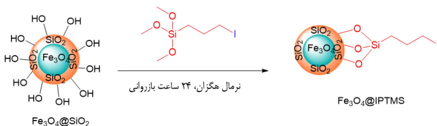
شکل ۳ طرحواره سنتز نانوذره های مغناطیسی Fe_3O_4@IPTMS
