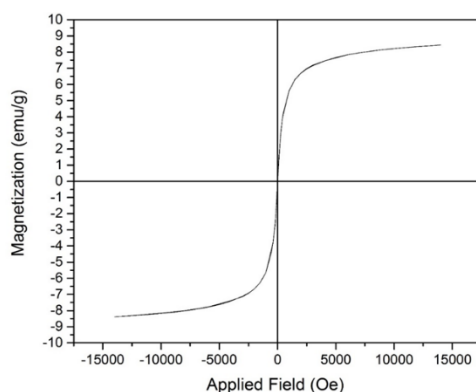
شکل ۱۳ نمودار VSM از نانوکاتالیست Fe 3 O 4 @PDBOA-Cu
