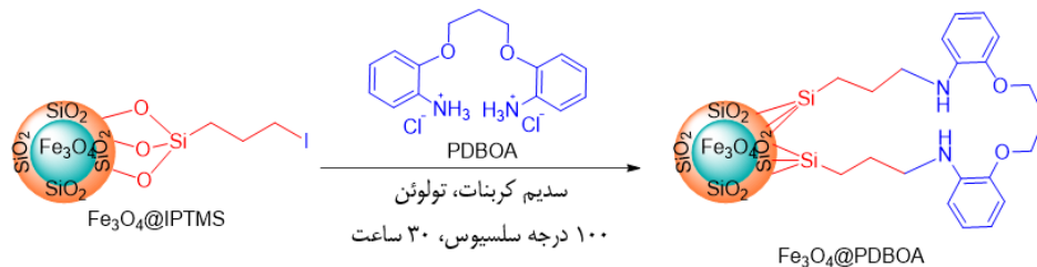
شکل ۴ طرح‌واره عامل‌دار کردن نانوذره‌های \text{Fe}_3\text{O}_4\text{@IPTMS} با لیگاند ۲ و ۱- (پروپان-۳-دی‌ایل-بیس(اکسی))دی‌آنیلین (PDBOA) برای سنتز \text{Fe}_3\text{O}_4\text{@PDBOA}
