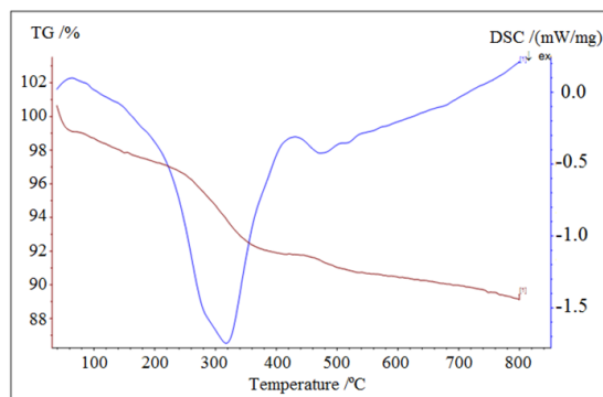
شکل ۱۲ نمودار TGA/DSC از نانوکاتالیست مغناطیسی Fe 3 O 4 @PDBOA-Cu
