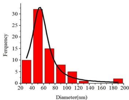
شکل ۸ نمودار بافت‌نگاشت برای تعیین توزیع اندازه ذره‌های نانوکاتالیست \text{Fe}_3\text{O}_4@\text{PDBOA-Cu}
