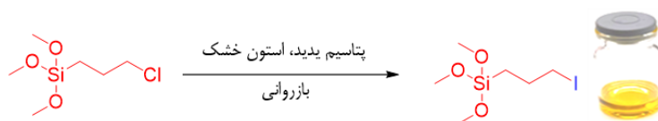
شکل ۲ طرحواره سنتز ۳-یدوپروپیل تری متوکسی سیلان (IPTMS)
