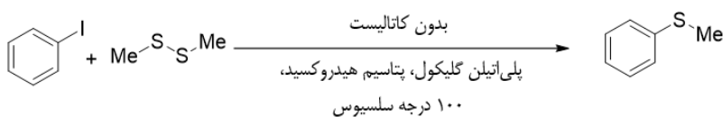
شکل ۱۵ طرح‌واره تبدیل دی‌متیل دی‌سولفید (DMDS) به متیل فنیل سولفید (MPS) در شرایط بدون کاتالیست
