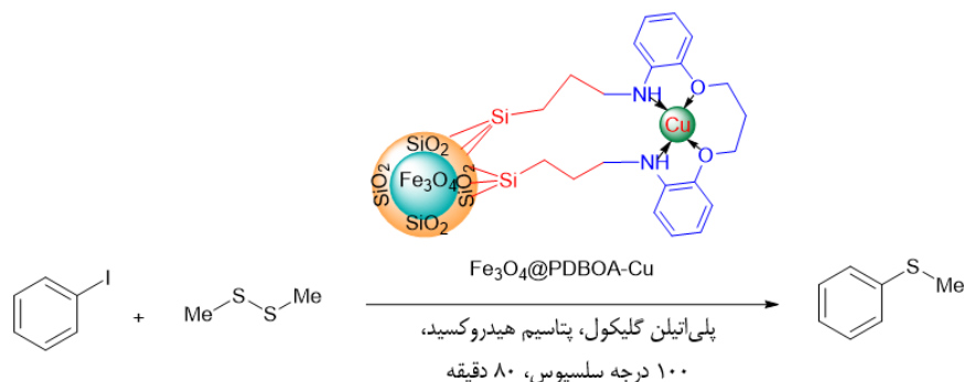
شکل ۶ طرحواره تبدیل DMS به MPS با نانوکاتالیست \text{Fe}_3\text{O}_4@\text{PDBOA}-\text{Cu}
