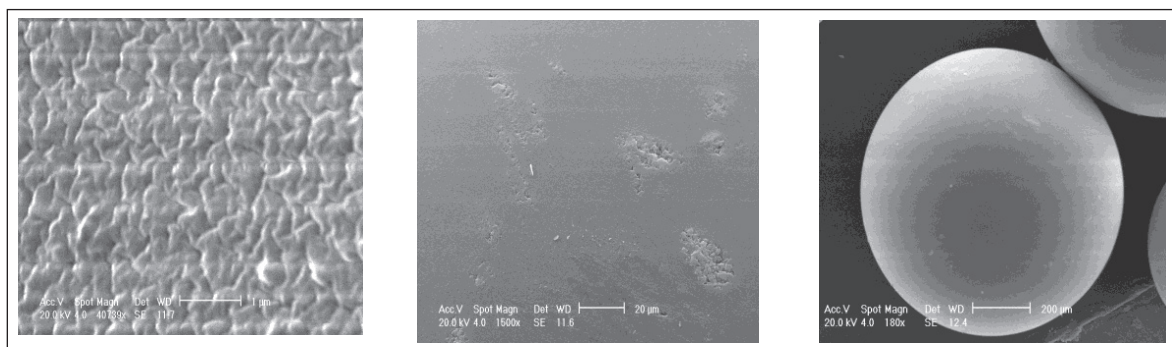
شکل ۲ تصویر SEM سطح رزین Amberlite XAD-4 شسته شده با آب و اتانول
