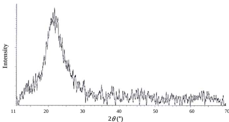
شکل ۳ الگوی پراش پرتو ایکس نانوذره های سنتز شده
