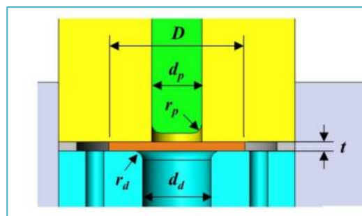
شکل (۳): پارامترهای مجموعه قالب [۱۸]
