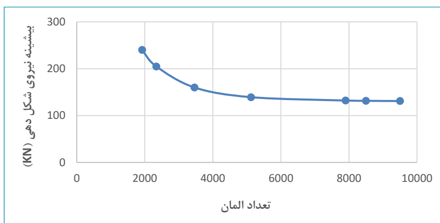
شکل ۴: تاثیر تعداد المان بر پیشینه نیروی شکل دهی [۱۶]
