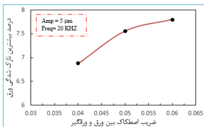
شکل ۱۲: منحنی نازک‌شدگی بر حسب ضریب اصطکاک ورق با ورق‌گیر
