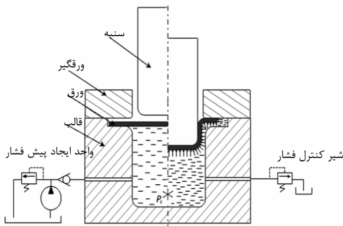
شکل ۱: فرایند کشش عمیق هیدرودینامیکی با فشار شعاعی [۴]
