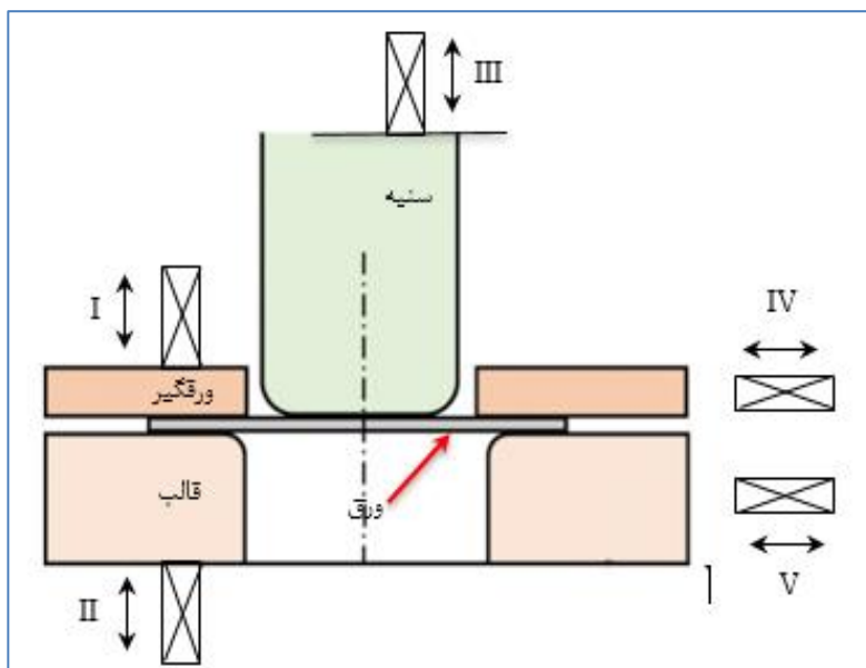
شکل ۲: روش‌های اعمال ارتعاش فراصوتی در فرایند کشش عمیق هیدرودینامیکی [۱۲]
