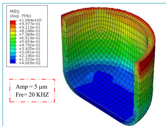
شکل ۱۰: قطعه شکل داده شده با فشار نهایی ۳۴ مگاپاسکل
