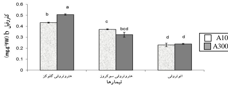
شکل ۵: هیستوگرام مقایسه محتوای کلروفیل b، بین تیمارها (A1300) و شاهد آنها (A10) در جلبک Chlorella vulgaris Beijernick.
