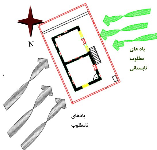
شکل ۴. جهت گیری بناها به سمت بادهای مطلوب تابستانی و محافظت در برابر بادهای نامطلوب زمستان
