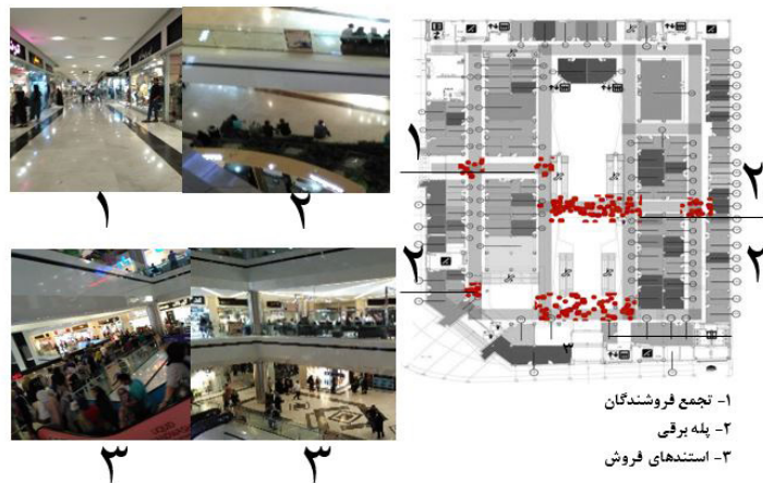
شکل ۶. مناطق پرازدحام طبقه همکف و اول
