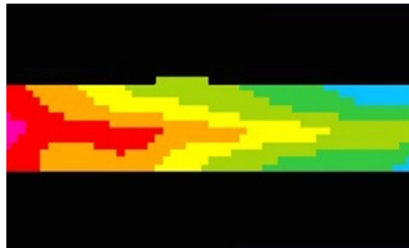
شکل ۹. کانتور دمای هوا
