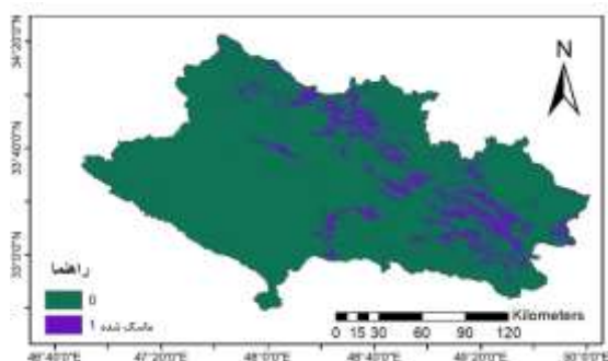
شکل ۶) تصویر آستانه گذاری شده و لایه ماسک شده جهت تخمین مساحت مناطق سیل زده استان لرستان طی روزهای ۲۰۱۹/۳/۲۰-۲۰۱۹/۴/۲۰ (منبع: نگارندگان)
