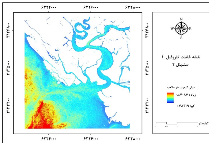
شکل ۵. نقشه غلظت کلروفیل - آ تهیه شده از الگوریتم OC2 سنتینل ۲-
