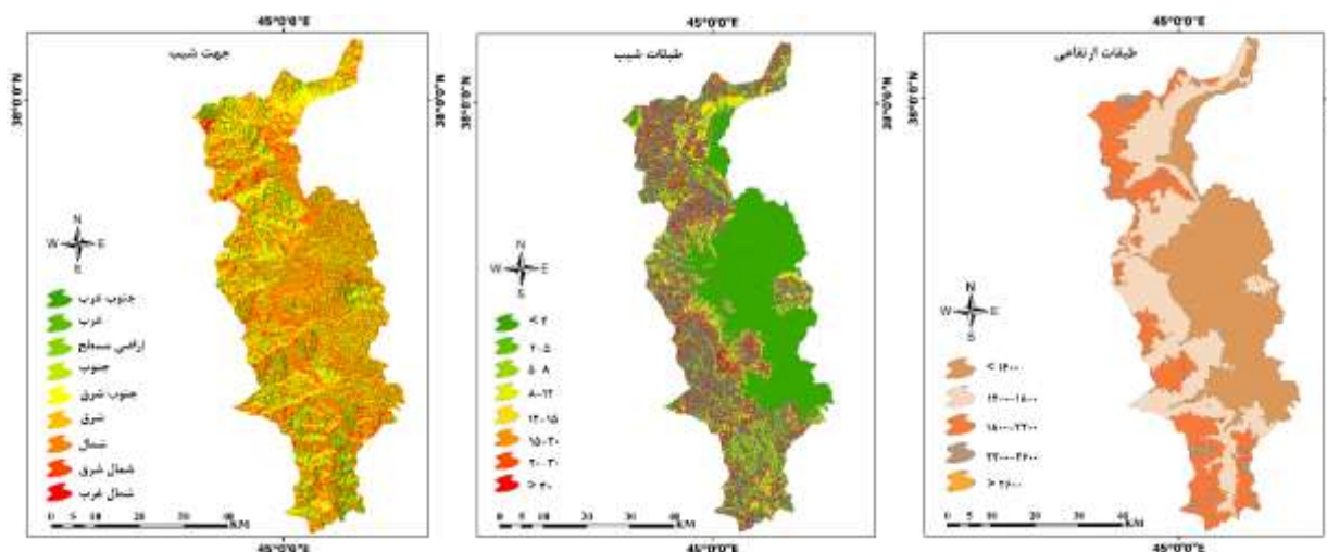
شکل (۲): نقشه طبقات ارتفاعی، طبقات شیب و جهت شیب در دشت ارومیه
