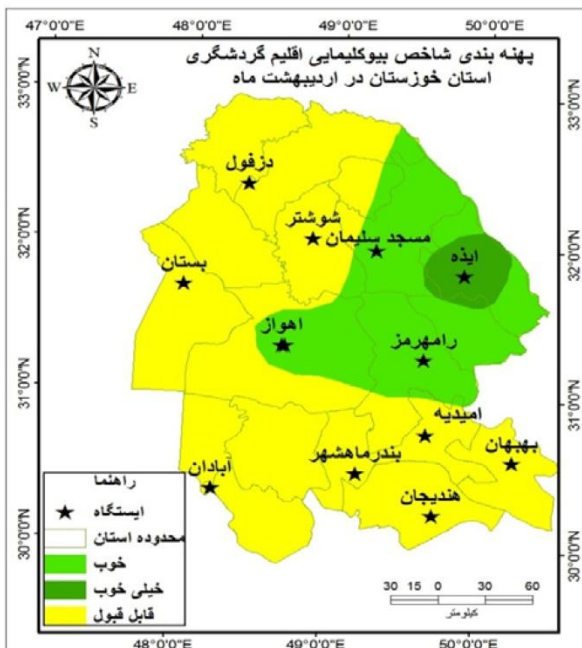
شکل ۲۷: پهنه بندی شاخص بیوکلیمایی اقلیم گردشگری اردیبهشت
