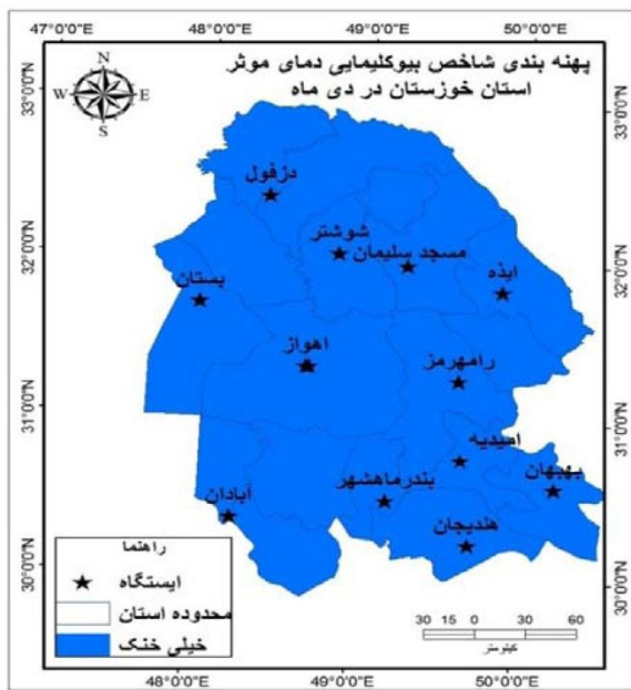
شکل ۲۳: شاخص بیوکلیمایی دمای موثر دی ماه
