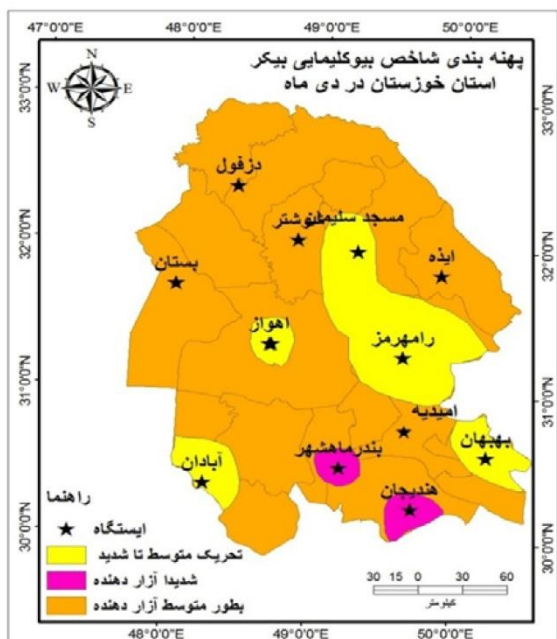
شکل ۱۰: شاخص بیوکلیمایی بیکر آذر ماه
