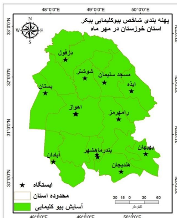
شکل ۸: شاخص بیوکلیمایی بیکر مهر ماه
