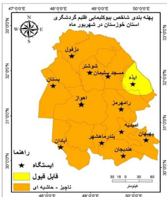
شکل ۳۱. پهنه بندی شاخص بیوکلیمایی اقلیم گردشگری شهر یور
