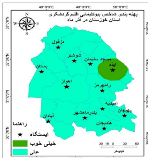
شکل ۳۴. پهنه بندی شاخص بیوکلیمایی اقلیم گردشگری آذر
