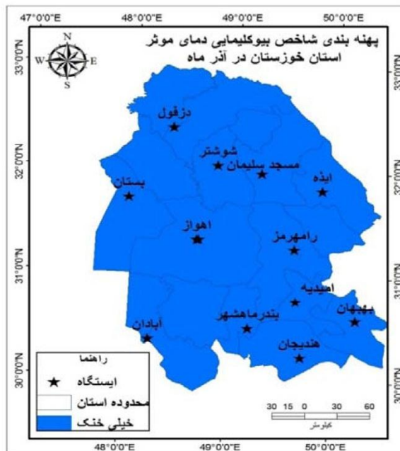
شکل ۲۲: شاخص بیوکلیمایی دمای موثر آذر ماه
