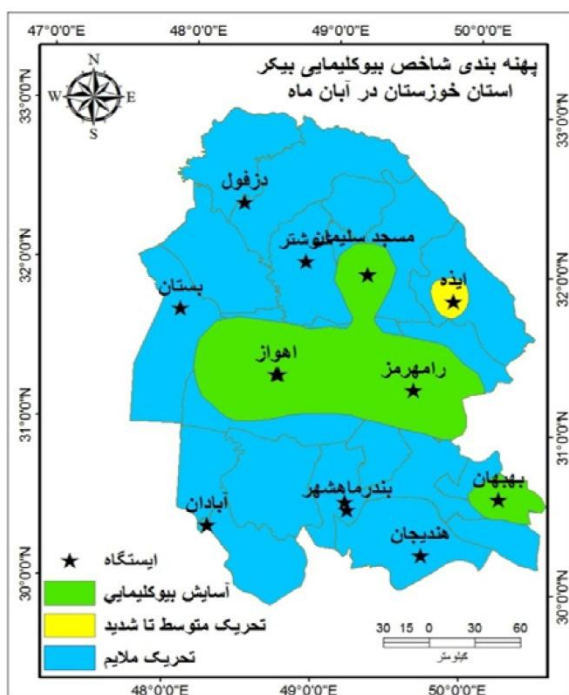
شکل ۹: شاخص بیوکلیمایی بیکر آبان ماه
