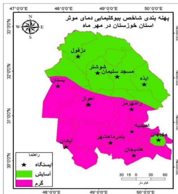
شکل ۲۰: شاخص بیوکلیمایی دمای مؤثر مهر ماه
