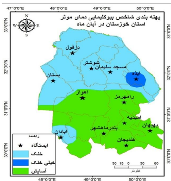
شکل ۲۱: شاخص بیوکلیمایی دمای مؤثر آبان ماه
