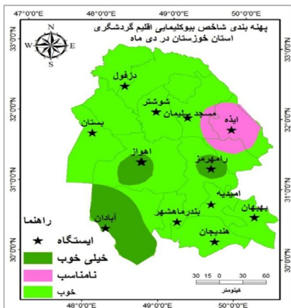
شکل ۳۵. پهنه بندی شاخص بیوکلیمایی اقلیم گردشگری دی
