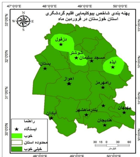
شکل ۲۶: پهنه بندی شاخص بیوکلیمایی اقلیم گردشگری فروردین
