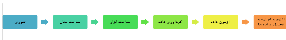
شکل شماره ۵ - مراحل اساسی اجرای تحلیل مدل بایبی معادلات ساختاری SEM (Human, 2009)
