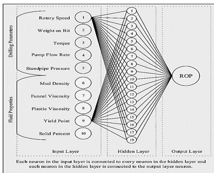
شکل ۱: شماتیک محاسبه سرعت نرخ نفوذ به روش شبکه فازی عصبی (Ahmed et al., 2019).
