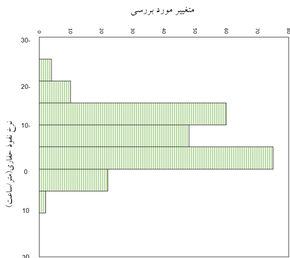
شکل ۵: هیستوگرام داده‌های نرخ نفوذ حفاری در برابر عمق حفاری، مدت زمان عملیات حفاری، سرعت گردش مته، وزن روی مته، وزن و حجم گل حفاری
