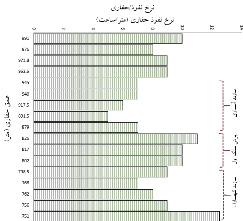
شکل ۴: نمودار نرخ نفوذ بر حسب عمق حفاری در سازندهای مختلف میدان ابودر
