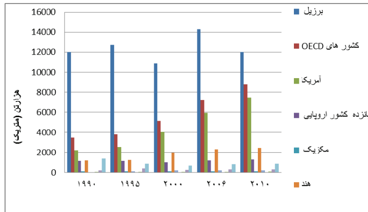
نمودار ۲- تولید جهانی اتانول
