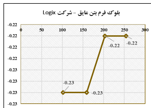
دیاگرام ۷ - تغییرات تعادل حرارتی بلوک شرکت Logix
