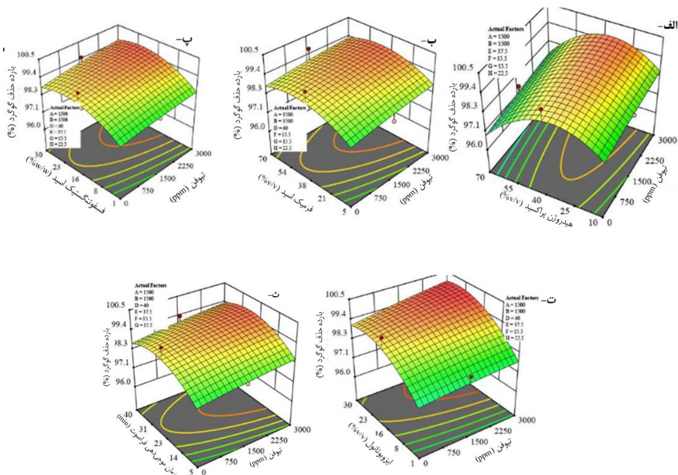
شکل ۴. تأثیر متقابل مقادیر مختلف ترکیب تیوفنی نسبت به بازده حذف گوگرد در نمونه سنتزی بر حسب (الف) هیدروژن پراکسید، (ب) فرمیک اسید، (پ) فسفونگستیک اسید، (ت) ایزو بوتانول، (ث) زمان.
