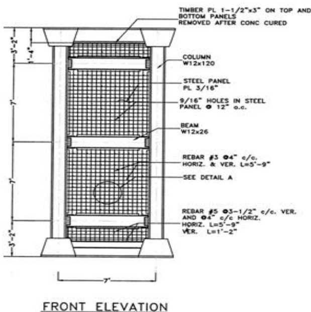
شکل ۲- نمایی از آرماتوربندی نمونه [۱]
