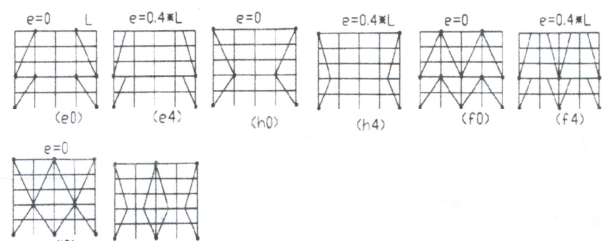
شکل ۹-۴: نمایش ابرباندنهای همگرا و واگرا در طرحهای تقویت نظیر گروههای e, f, h, i
