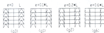
شکل ۱۰-۵: گروه g با باندنهای همگرا و واگرای متداول برای تقویت لرزه ای قاب مورد بررسی
