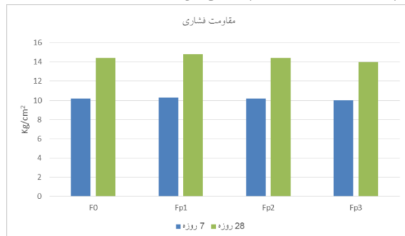
شکل ۶- مقاومت فشاری طرح‌های حاوی الیاف پلی پروپیلن
