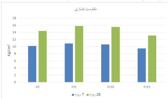
شکل ۸- مقاومت فشاری طرح‌های حاوی خاکستر شلتوک برنج
