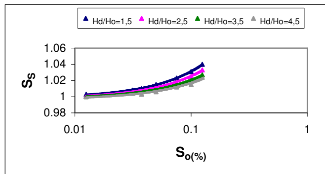
شکل ۱۴- ضریب تصحیح مربوط به شیب کف لایه آبدار
