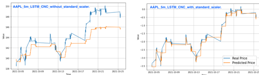
شکل (۷) پیش‌بینی قیمت پایانی برای AAPL فهرست‌شده در NASDAQ با استفاده از 1D CNN و LSTM برای مقایسه داده‌های استاندارد‌شده و غیر استاندارد در بازه زمانی ۵ دقیقه
