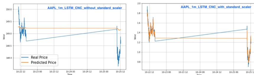
شکل (۶) پیش‌بینی قیمت پایانی برای AAPL فهرست‌شده در NASDAQ با استفاده از 1D CNN و LSTM برای مقایسه داده‌های استاندارد شده و غیر استاندارد در بازه زمانی ۱ دقیقه
