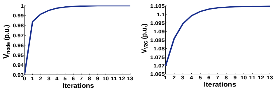
(الف) ولتاژ شین تجميع کننده خودروهای برقی (ب) ولتاژ شین اتصال تجميع کننده خودروهای برقی به شبکه
