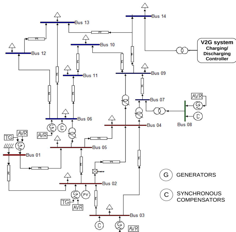
شکل (۵): سیستم توزیع ۱۴ باسه مجهز به تکنولوژی خودروی برقی به شبکه
