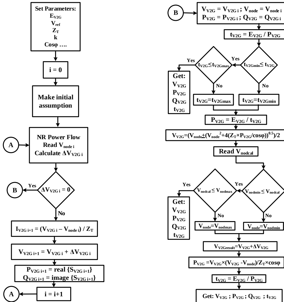
شکل (۴): فلوچارت روش پیشنهادی برای کنترل کننده شارژ-دشارژ سیستم خودروی برقی به شبکه
