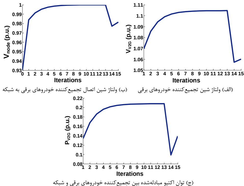
شکل (۸): ولتاژ و توان اکتیو مبادله شده بین تجميع کننده خودروهای برقی و شبکه در سناریوی سوم
