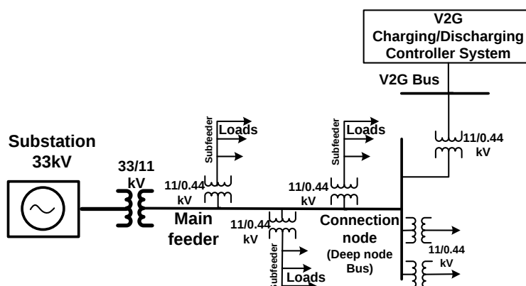
شکل (۳): سیستم توزیع شعاعی نمونه [۱۶]
