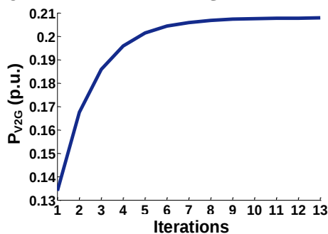
(ج) توان اکتیو مبادله شده بین تجميع کننده خودروهای برقی و شبکه
