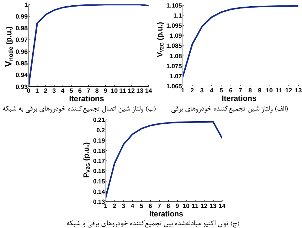
شکل (۷): ولتاژ و توان اکتیو مبادله شده بین تجميع کننده خودروهای برقی و شبکه در سناریوی دوم
