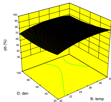
شکل ۸- بررسی اثر متقابل دما و تراکم بر میزان جذب سرب در جلبک کلرلا در روش تولید بیوفیلم
