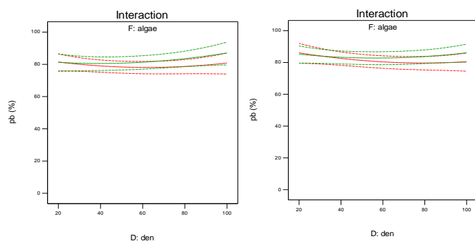
شکل ۱۳- بررسی اثر متقابل تراکم و نوع جلبک بر میزان جذب سرب در روش بیوفیلم (سمت راست) و سوسپانسیون (سمت چپ)
