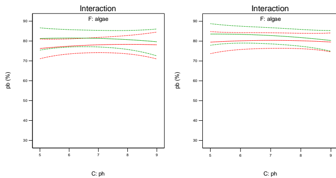
شکل ۲- تأثیر pH بر میزان جذب سرب توسط میکروجلبک‌ها در دو روش تولید بیوفیلیم (سمت راست) و سوسپانسیون (سمت چپ)
