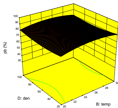
شکل ۹- بررسی اثر متقابل دما و تراکم بر میزان جذب سرب در جلبک سندسموس در روش تولید بیوفیلم
