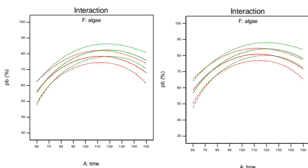
شکل ۶- تأثیر زمان تماس با جاذب بر جذب فلز سنگین سرب در دو روش تولید بیوفیلم (سمت راست) و سوسپانسیون (سمت چپ)
