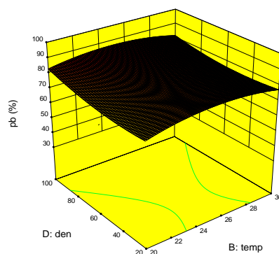
شکل ۱۱- بررسی اثر متقابل دما و تراکم بر میزان جذب سرب در جلبک سندسموس در روش تولید سوسپانسیون
