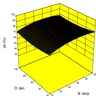
شکل ۱۰- بررسی اثر متقابل دما و تراکم بر میزان جذب سرب در جلبک کلرلا در روش تولید سوسپانسیون
