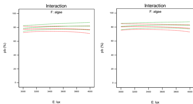
شکل ۱۵- بررسی اثر متقابل شدت نور و نوع جلبک بر میزان جذب سرب در روش بیوفیلم (سمت راست) و سوسپانسیون (سمت چپ)
