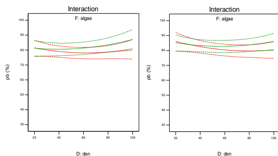
شکل ۵- تاثیر تراکم فلز سنگین بر میزان جذب سرب در دو روش تولید بیوفیلم (سمت راست) و سوسپانسیون (سمت چپ)
