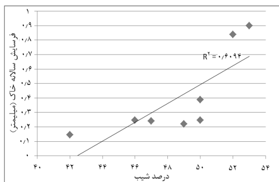
شکل ۵- نمودار فرسایش خاک و درصد شیب
