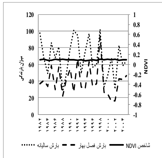
شکل ۴- تغییرات شاخص NDVI و بارندگی در منطقه کشاورزی
