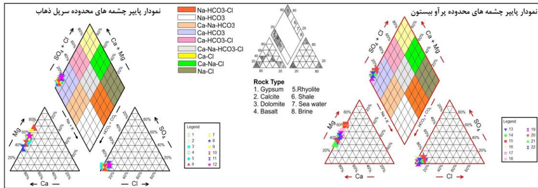
شکل ۳: نمودار پایپر چشمه‌های آبخوان بیستون و آبخوان‌های سریل ذهاب
