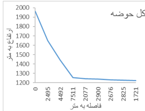
شکل ۴: نیمرخ طولی رودخانه کرج (بالادست مهرشهر)
