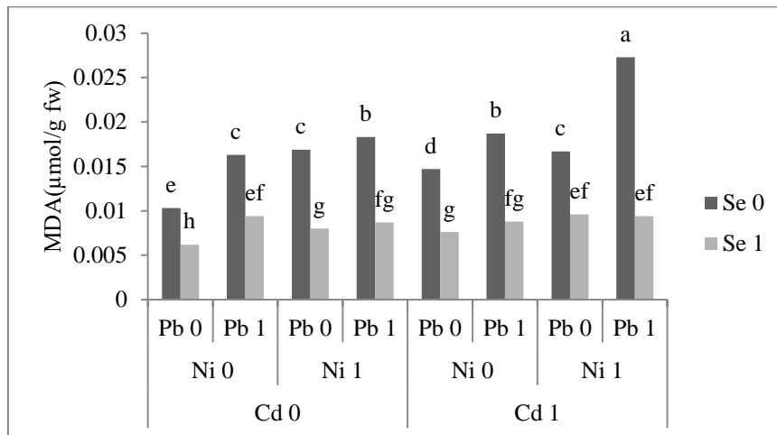
شکل ۳: اثر سلنیوم (Se) بر محتوای مالون دی آلدئید (MDA) گیاهچه خیار تحت تنش همزمان عناصر سنگین کادمیوم (Cd)، نیکل (Ni) و سرب (Pb)
