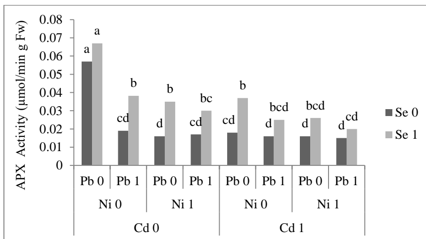
شکل ۶: اثر سلنیوم (Se) بر فعالیت آنزیم آسکوربات پراکسیداز (APX) در گیاهچه خیار تحت تنش همزمان عناصر سنگین کادمیوم (Cd)، نیکل (Ni) و سرب (Pb)
