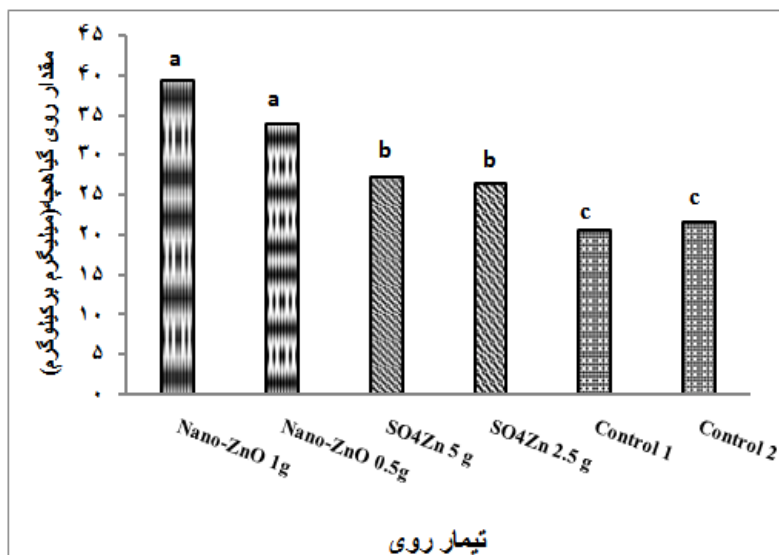
شکل ۲: تأثیر تیمار کردن بذر با کود روی بر مقدار روی گیاهچه
