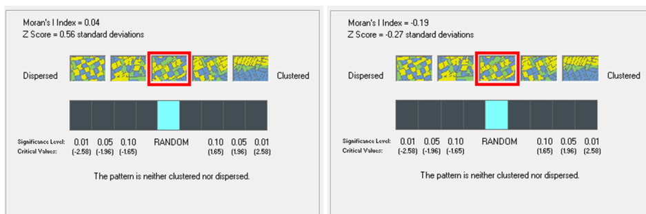
شکل (۴): الگوی پراکنش مراکز انتظامی در نواحی شهر یزد با استفاده از ضریب موران از روش صفر و یک و روش مرز مشترک
