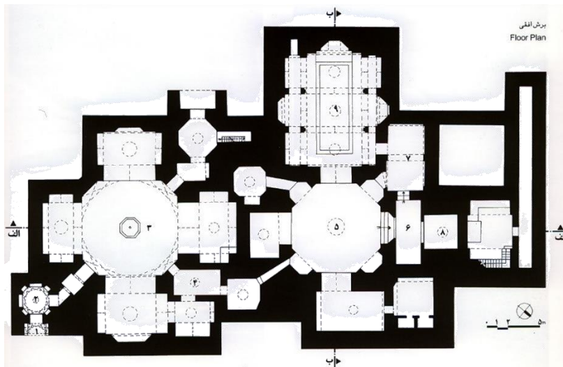
۱. ورودی ۲. هشتی ۳. بینه ۴. میان‌در ۵. گرم‌خانه ۶. خزینه ۷. شاه‌نشین ۸. تیان ۹. چال‌حوض. تصویر ۱. پلان حمام ایرانی (حمام شاه اصفهان)؛ مأخذ: گنج‌نامه.
