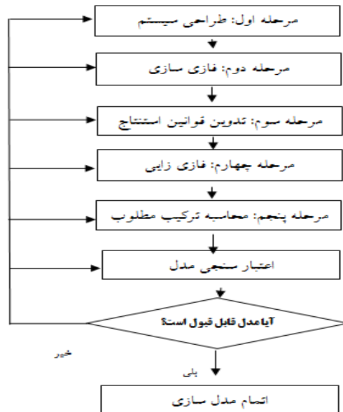
شکل شماره (۱) - الگوریتم مدل‌سازی
