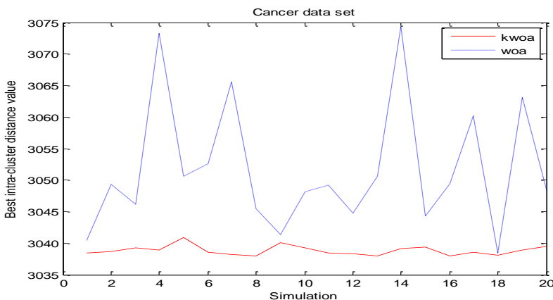
شکل شماره ۳: اجرای الگوریتم ترکیبی جدید و الگوریتم نهنگ روی داده cancer
