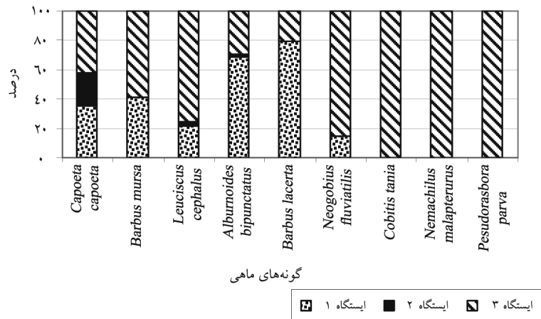
شکل ۴- درصد فراوانی گونه‌های مختلف ماهیان در ایستگاه‌ها، سال ۸۳-۱۳۸۲
