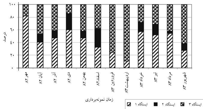
شکل ۳- درصد فراوانی ماهیان در ماه‌های مختلف نمونه برداری، سال ۸۳-۱۳۸۲
