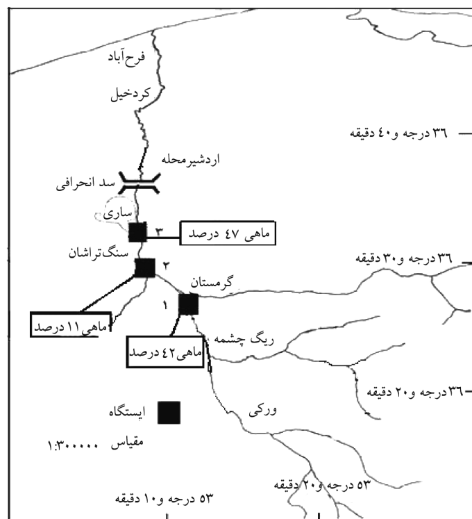
شکل ۱- حوضه آبریز رودخانه تجن، ایستگاه‌های نمونه‌برداری و درصد فراوانی سالانه ماهی
