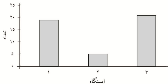
شکل ۲- میانگین سالانه تعداد ماهیان رودخانه تجن در ایستگاه‌ها ۸۳-۱۳۸۲
