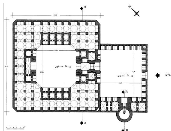
تصویر ۱۸: پلان رباط طرق (منبع: میراث فرهنگی خراسان رضوی).
