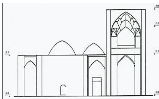
تصویر ۱۴: نمای شمال غربی رباط خیرآباد (منبع: میراث فرهنگی خراسان رضوی).
