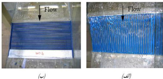
شکل 3: نمایی از شکل هندسی مدل فیزیکی
