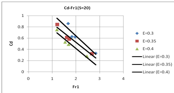
شکل 8: مقایسه ضریب C_d نسبت به عدد فرود به ازاء شیب 20 درجه
