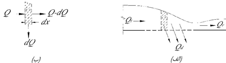
شکل 2: (الف) جریان بر روی یک آبگیر کفی، (ب) جریان در یک المان
